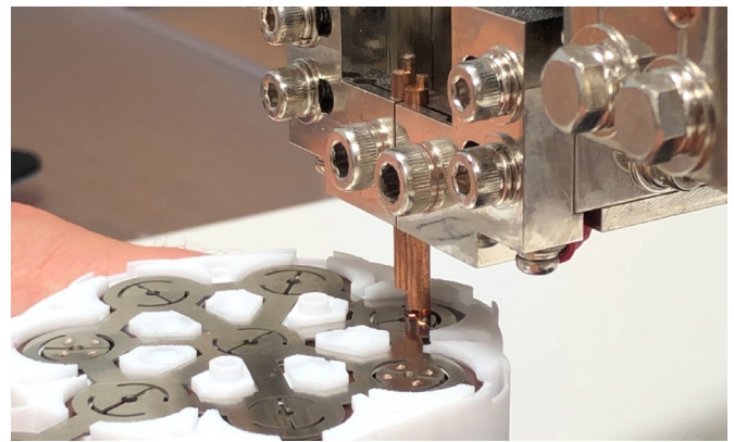
Neues Design der Stromverbinder
